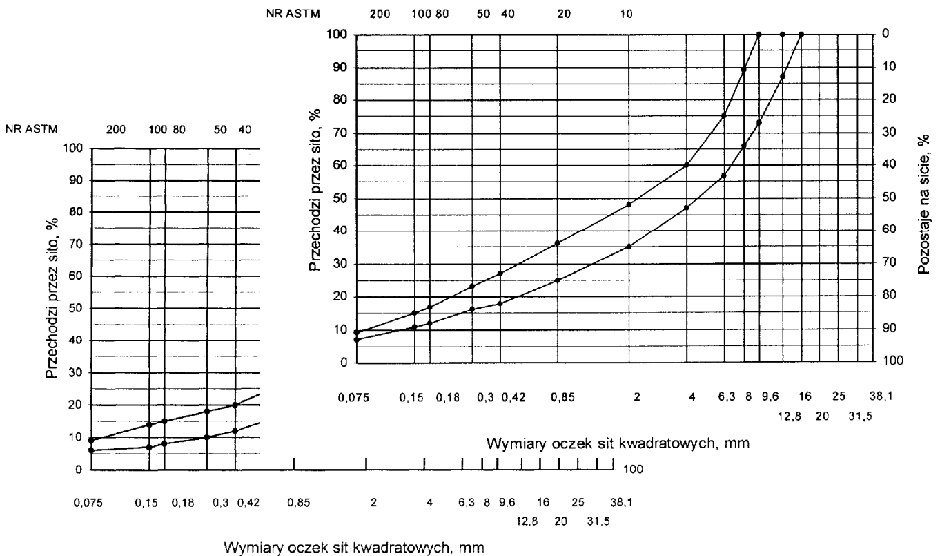
Rys. 7. Krzywe graniczne uziarnienia mieszanki mineralnej BA od 0 do 12,8 mm do warstwy ścieralnej nawierzchni drogi o obciążeniu ruchem od KR3 do KR6
